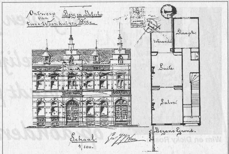
Bouwtekening uit 1895, het hoogtepunt van de Neo-rennaissance in Nijmegen. Deze tekening werd gebruikt bij de aanvraag van een vergunning om te bouwen aan de Berg- en Dalseweg. Het betreft hier twee maal een boven en een benedenwoning.
